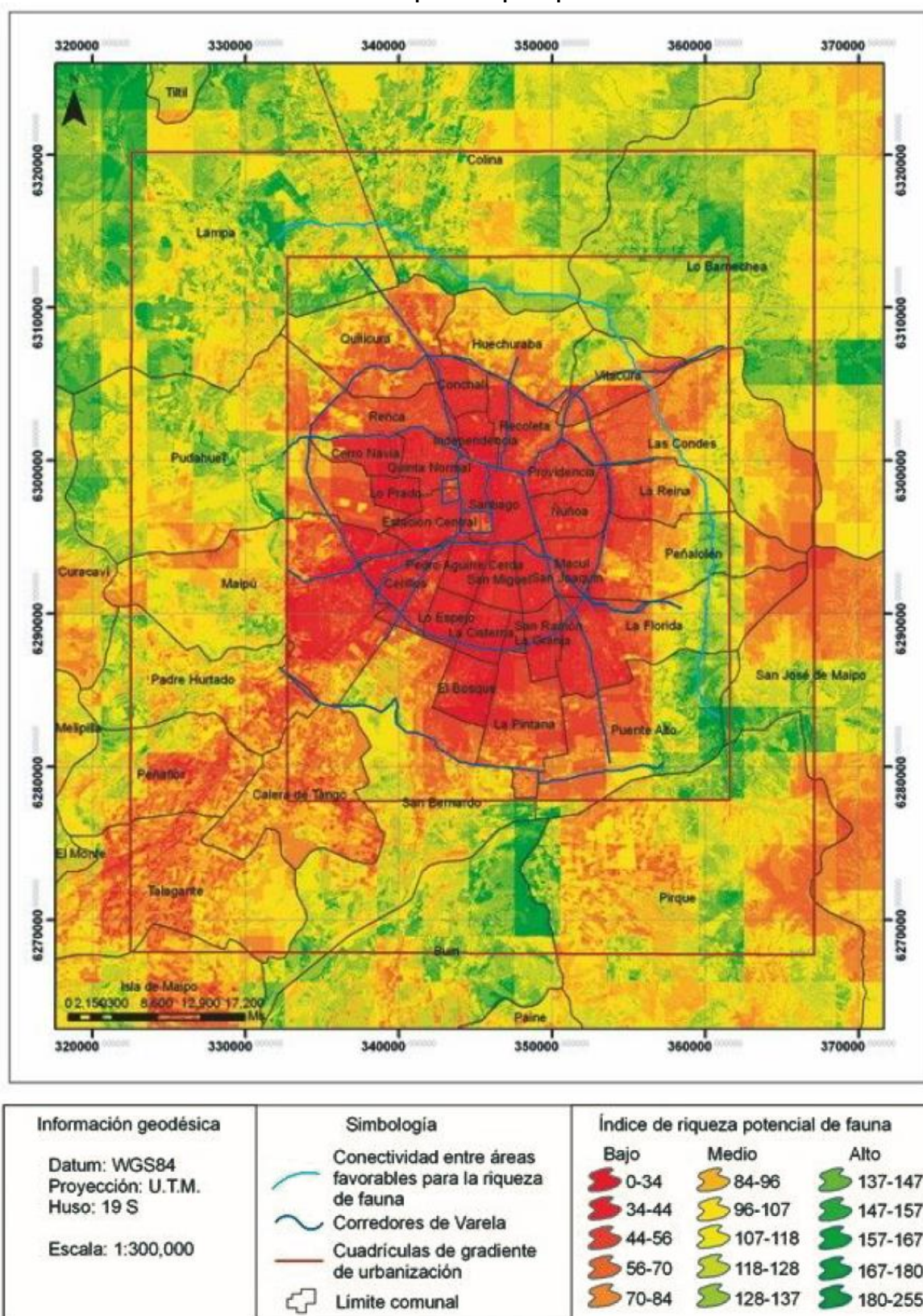
Ilustración 3-4 Áreas favorables para la riqueza potencial de fauna vertebrada
