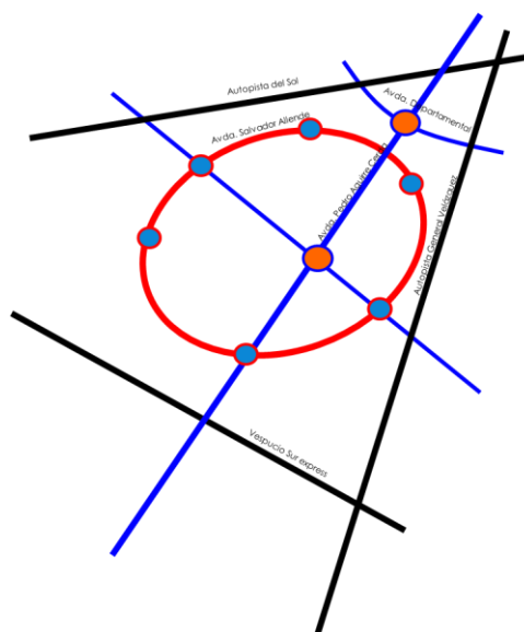
Figura 51: Esquema estructura general Alternativa 1
