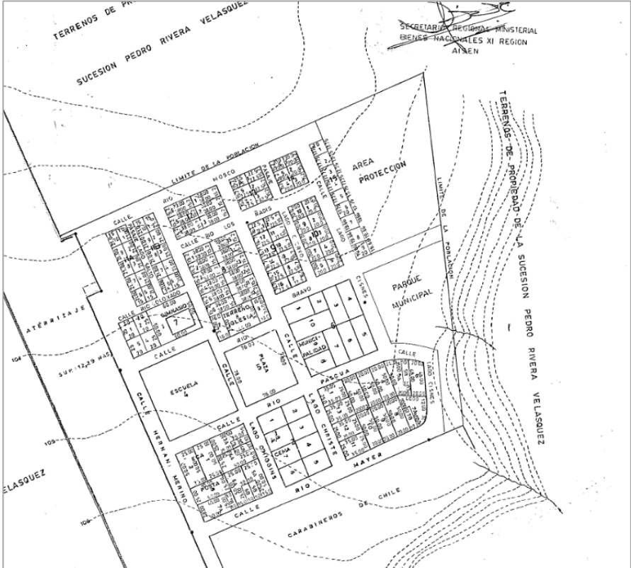
Imagen 4 Plano de loteo Villa O´ Higgins 1993
