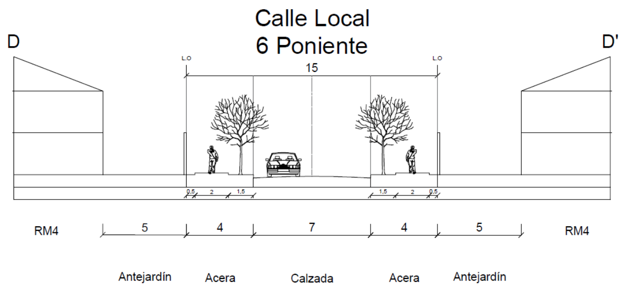
Imagen 62 Ejemplo de perfil para vía local propuesta de 15 m.
