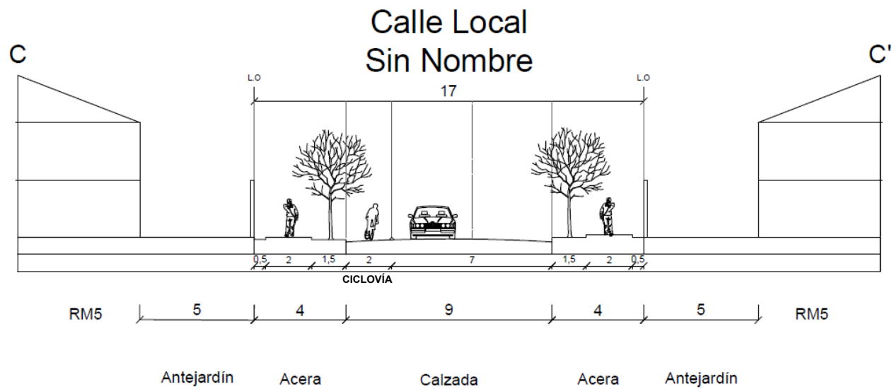
Imagen 61 Ejemplo de perfil para vía local propuesta de 17 m.
